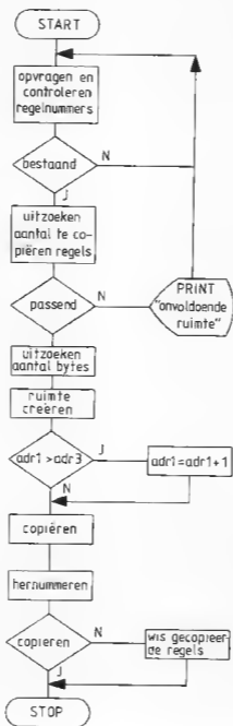
Afb. 10-1 Flow chart van het programma 'copymove'
